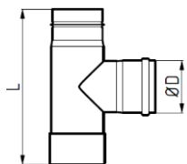
T - Stück / 250 mm lang / mit Kapsel
