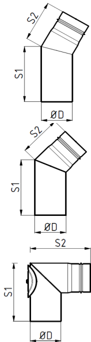
Bogen / 2-teilig / eingezogen
